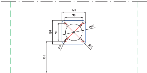
Gambone regolabile “ONG”. Colori disponibili vedi pag.23
