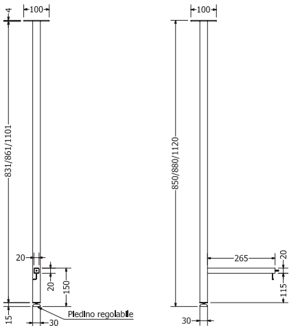
Schemi foratura per fissaggio Drilling diagrams for fixing
