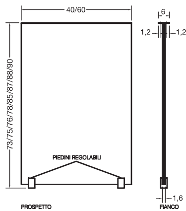
Disegno tecnico Technical drawing
